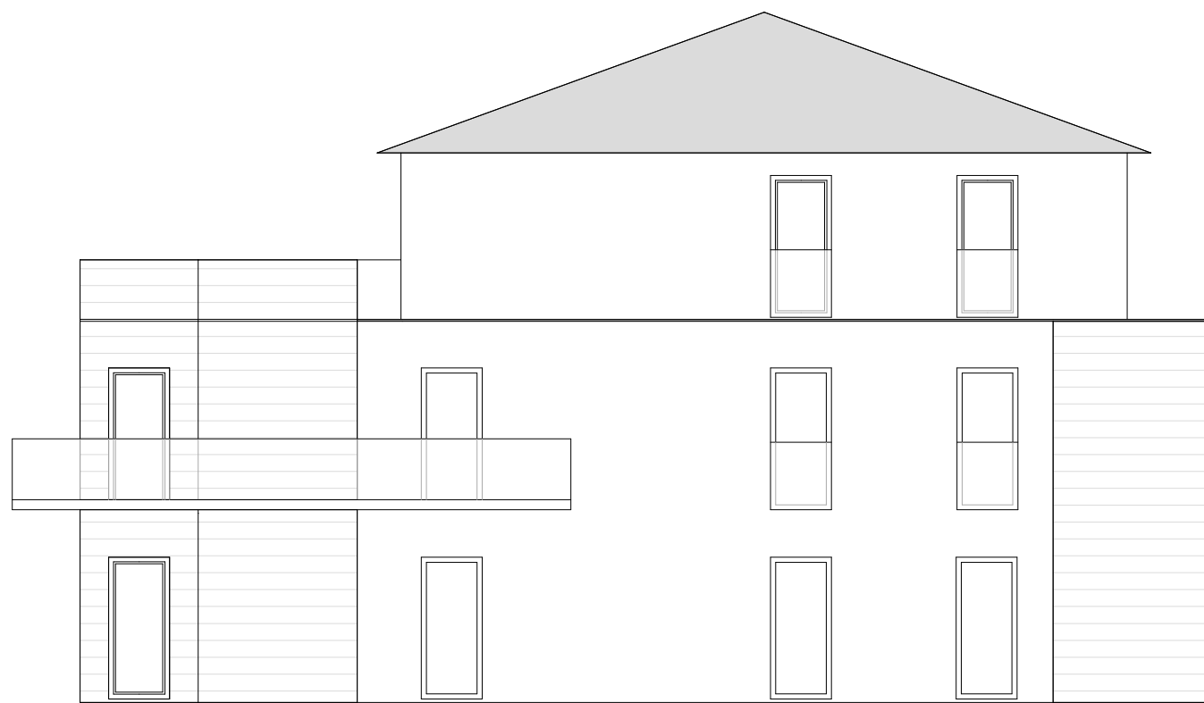
Ansicht Süd
