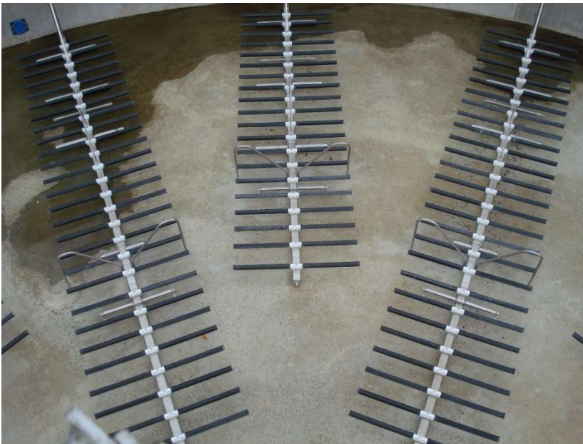
vorhandene Strangentlüfter 2014
